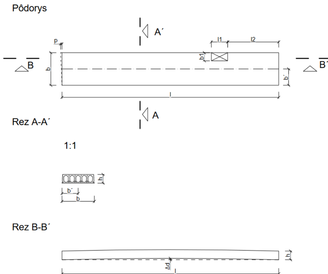
Obr.č.1 schéma odchýlok na paneloch
